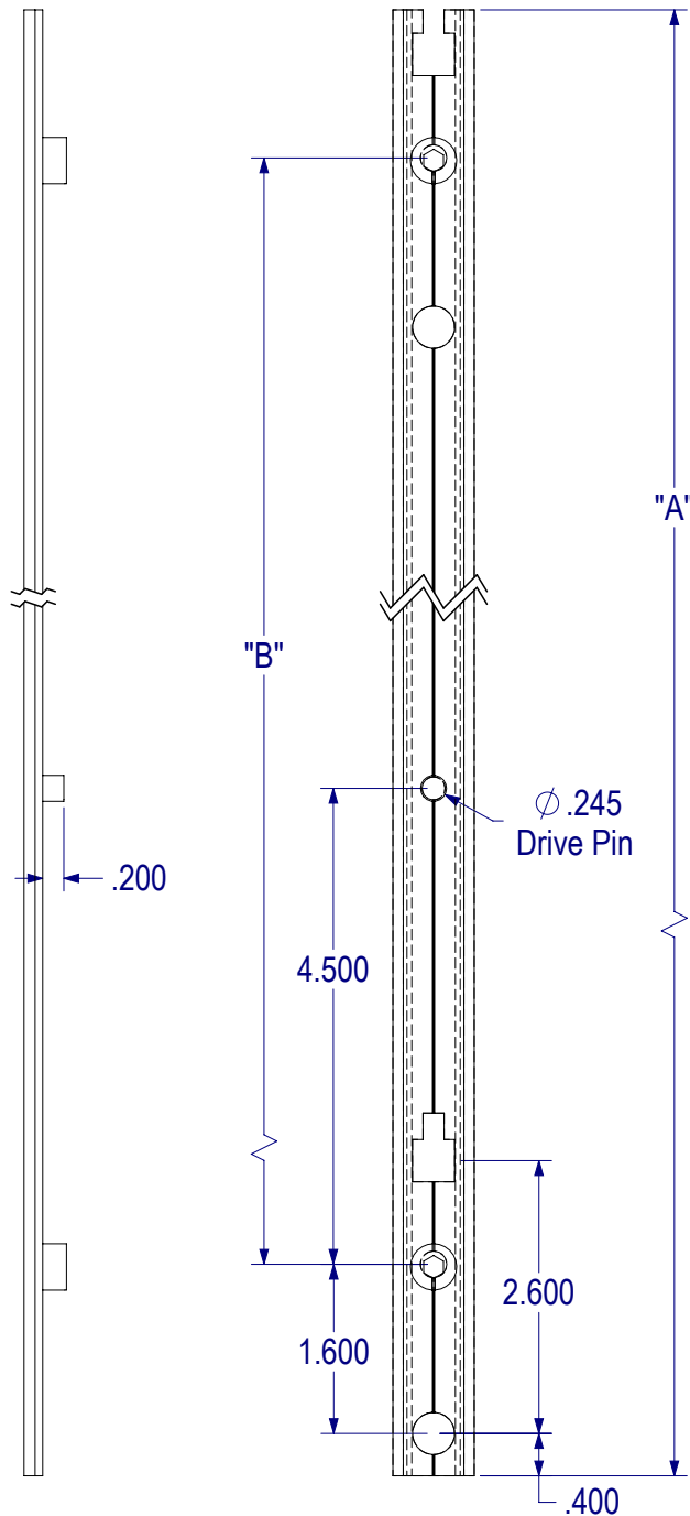
8039 Lock Bar
