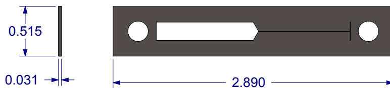
#8205 Gasket
